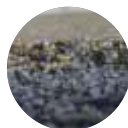
Nalożenie pierwszej warstwy TopStone
